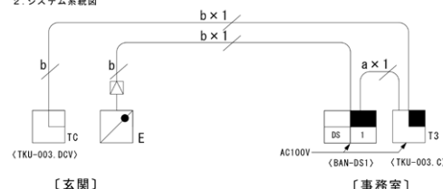
2. システム系統図
